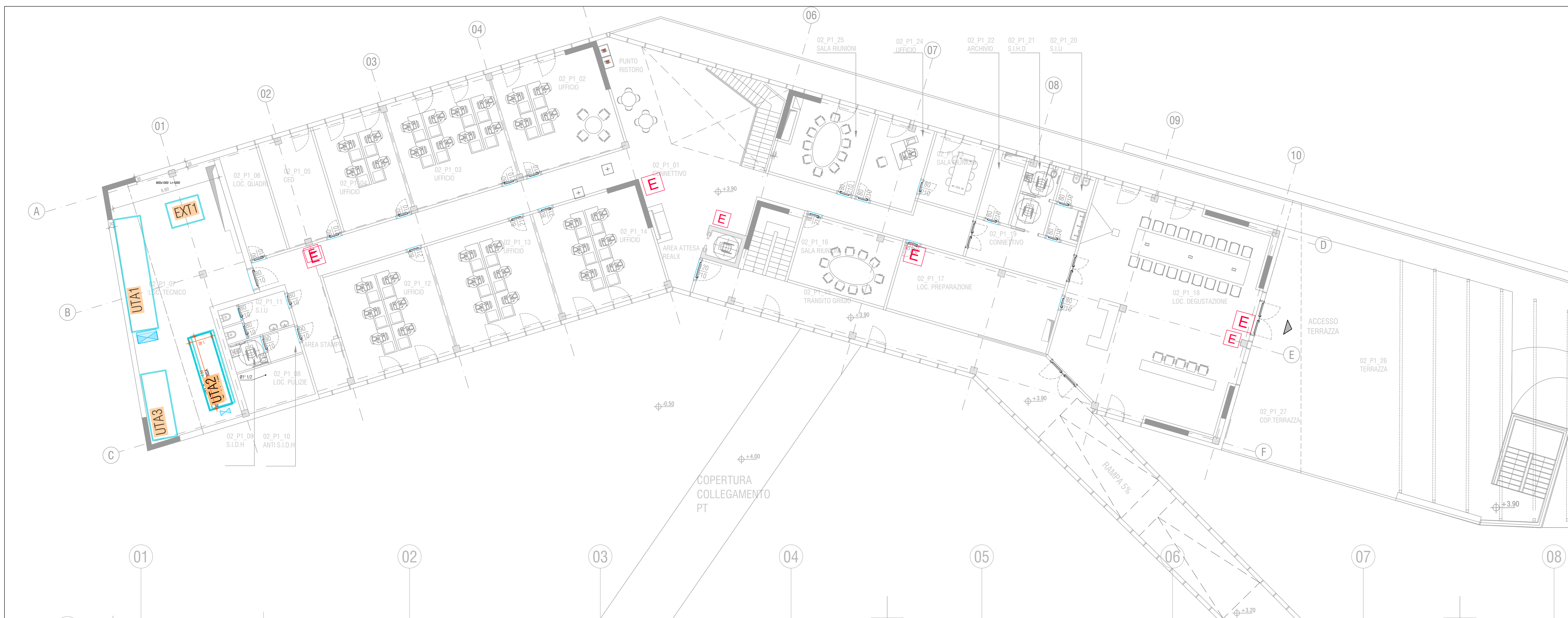
PIANTA PIANO PRIMO - DOTAZIONI ANTINCENDIO - SCALA 1:100
